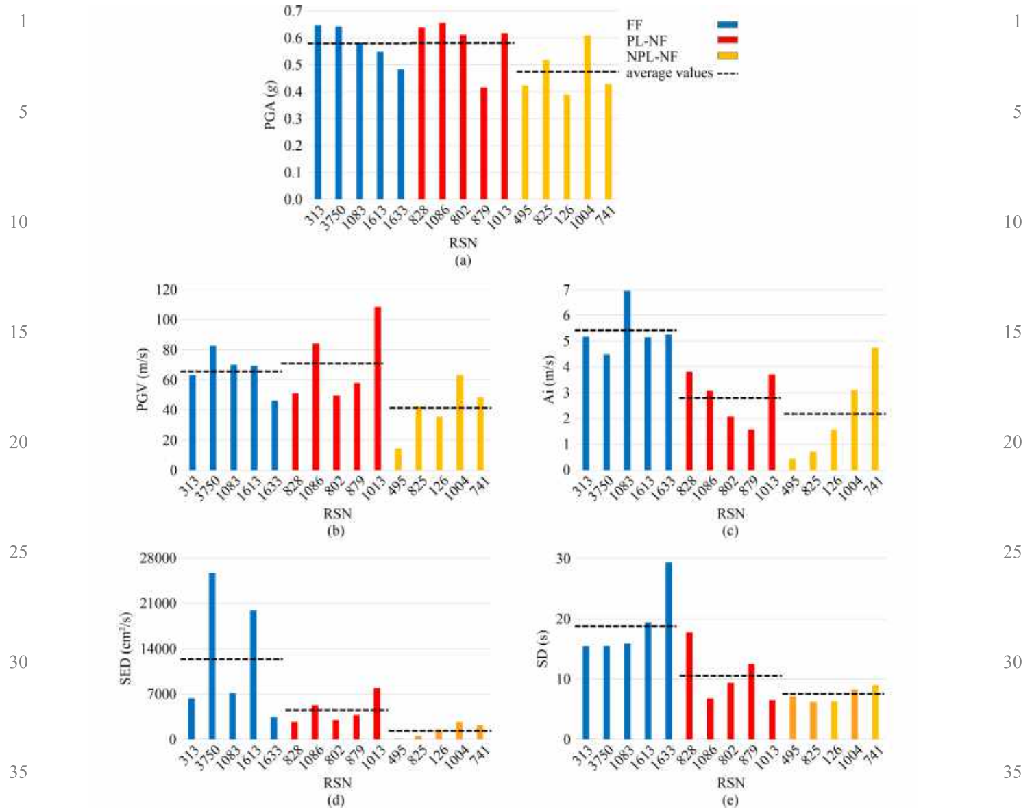
Fig. 10 Scaled seismic event records: (a) PGA ; (b) PGV ; (c) A_i ; (d) SED ; (e) SD .
